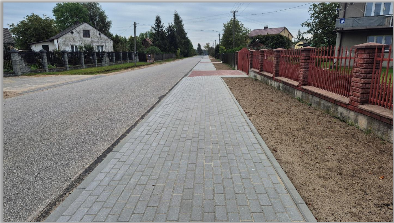
Przebudowa drogi powiatowej nr 2229W Jędrzejów – Ceglów – Kuflew polegająca na budowie chodnika od km 10+674 do km 11+025 (351 mb), m. Podskwarne
